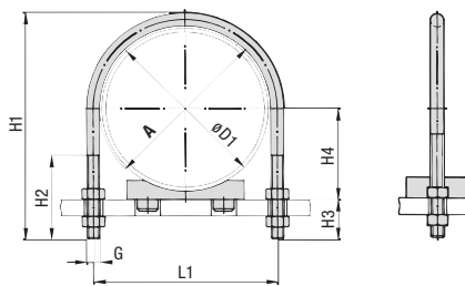
Rundstahlbügel (Typ RB) mit Kunststoff-Rohrauflege (Typ RUK)
