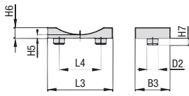
Kunststoff-Rohrauflage (Typ RUK) (bei Baugröße DN 40 ist das Maß L4 um 90° versetzt)
